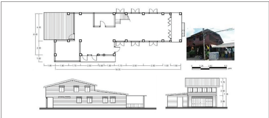
ภาพที่ 9: บ้านยาวโกย ผังพื้นและรูปตัด
