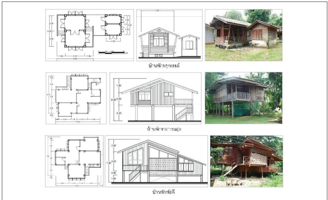
ภาพที่ 12: บ้านพักข้าราชการ
