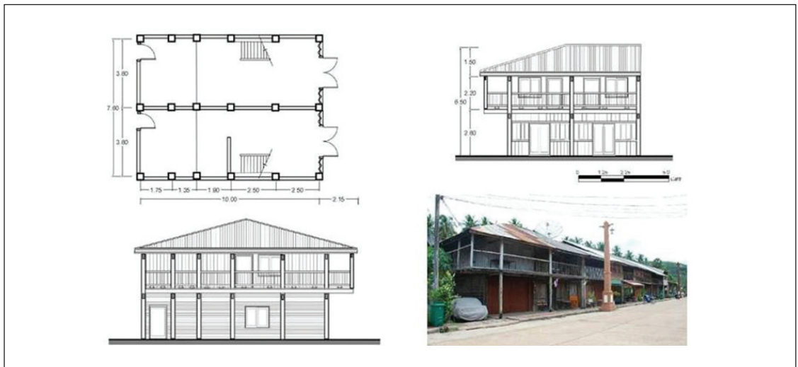
ภาพที่ 11: บ้านยาวสองช่วงเสา ผังพื้นและรูปตัด
