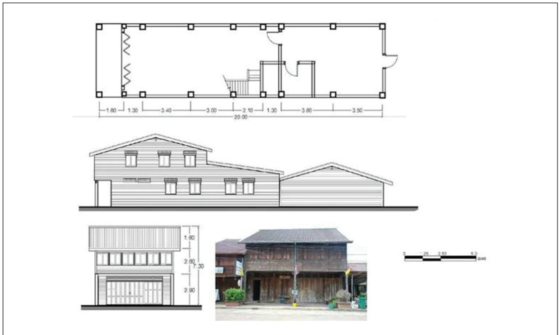
ภาพที่ 10: บ้านยาวหนึ่งช่วงเสา ผังพื้นและรูปตัด
