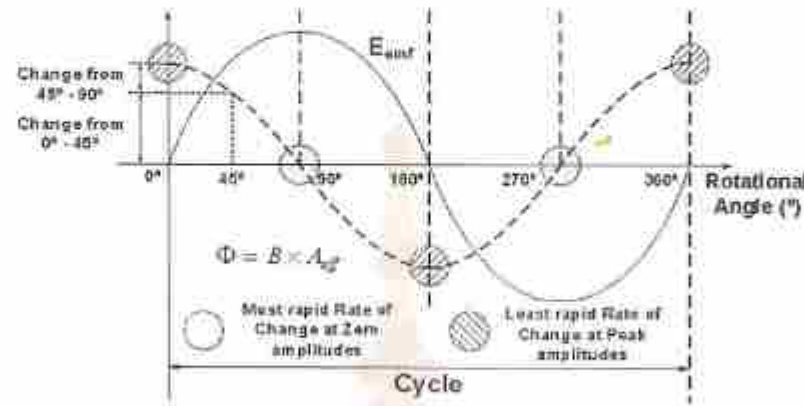
รูปที่ 2.4 ความต่างศักย์ของแหล่งกำเนิดไฟฟ้ากระแสสลับ (AC source) มีลักษณะเป็นรูป sine และ T คือ เวลาที่ครบ 1 รอบของสัญญาณ (ที่มา: macao.communications.museum)
