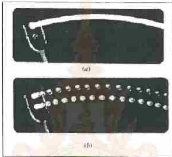
รูปที่ 2.12 แสดงภาพที่เห็นของ LED เมื่อแคว่งวงจรไปมา รูป (a) เมื่อแผง LED ต่อเข้ากับแหล่งจ่ายไฟฟ้ากระแสตรง และ (b) เมื่อแผง LED ต่อเข้ากับแหล่งจ่ายไฟฟ้ากระแสสลับ
