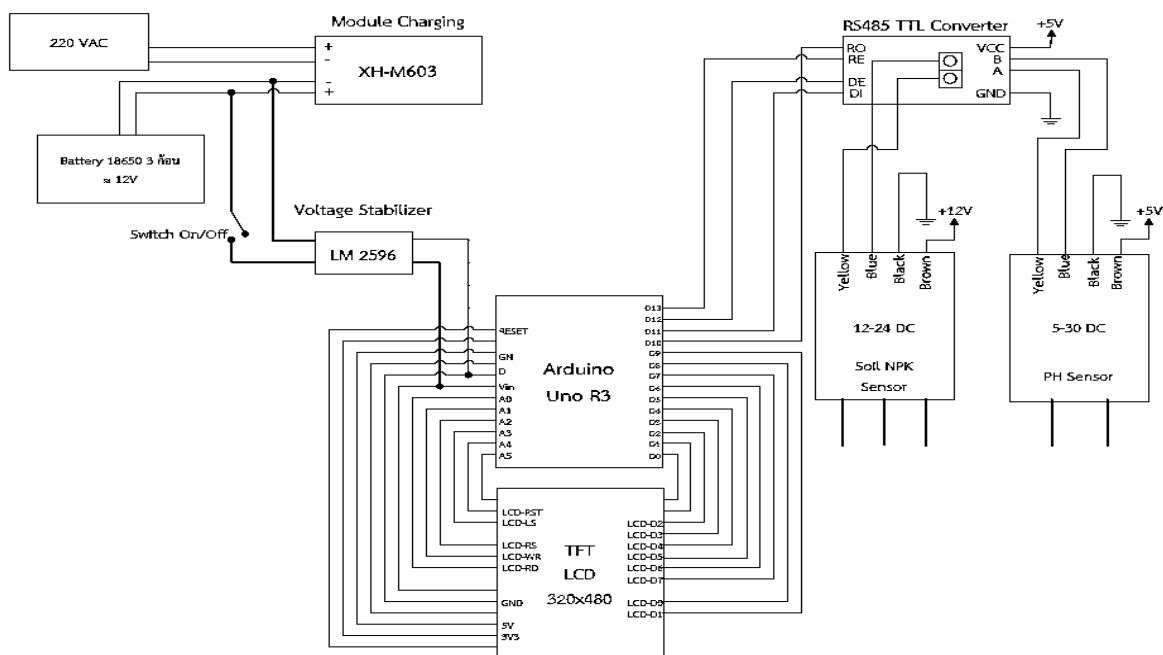
รูปที่ 1 การออกแบบการเชื่อมต่อเครื่องวิเคราะห์ค่าความเป็นกรดต่างและสารอาหารในดิน
