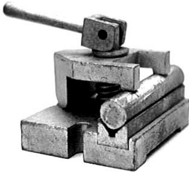
เครื่องมือจับยึดชิ้นงานทรงกระบอก (Clamping Device for a Cylindrical Workpeice)
