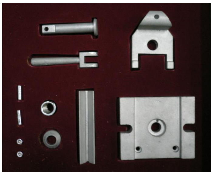
ถอดแยกชิ้นเครื่องมือจับยึดชิ้นงานทรงกระบอก
