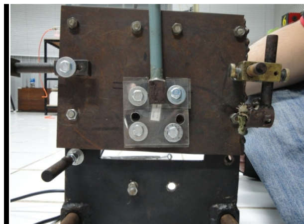
รูปที่ ข.9 ชุดวัดความดันจากการกระแทก
